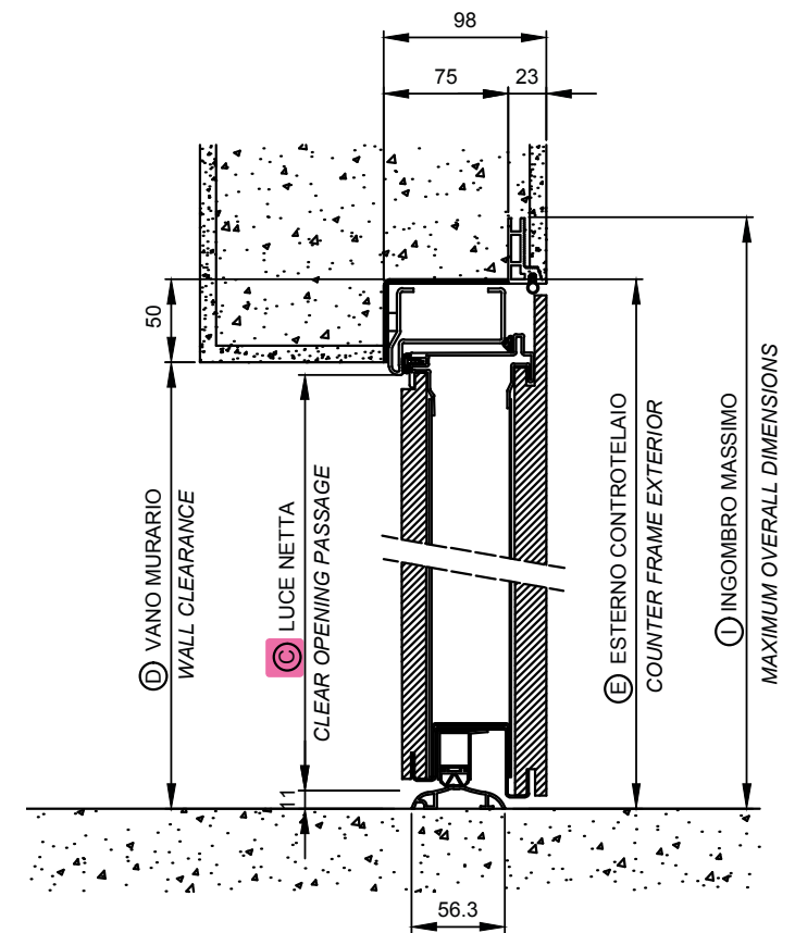
Configurazione con soglia tenuta aria-acqua-vento Configuration with air-water-wind tightness sill
