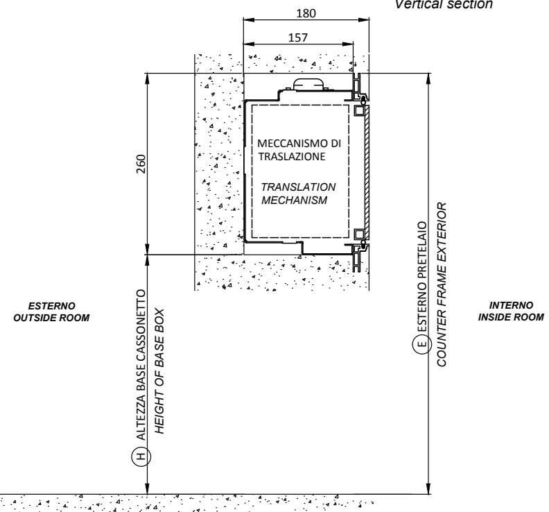
Sezione verticale D-D Vertical section
