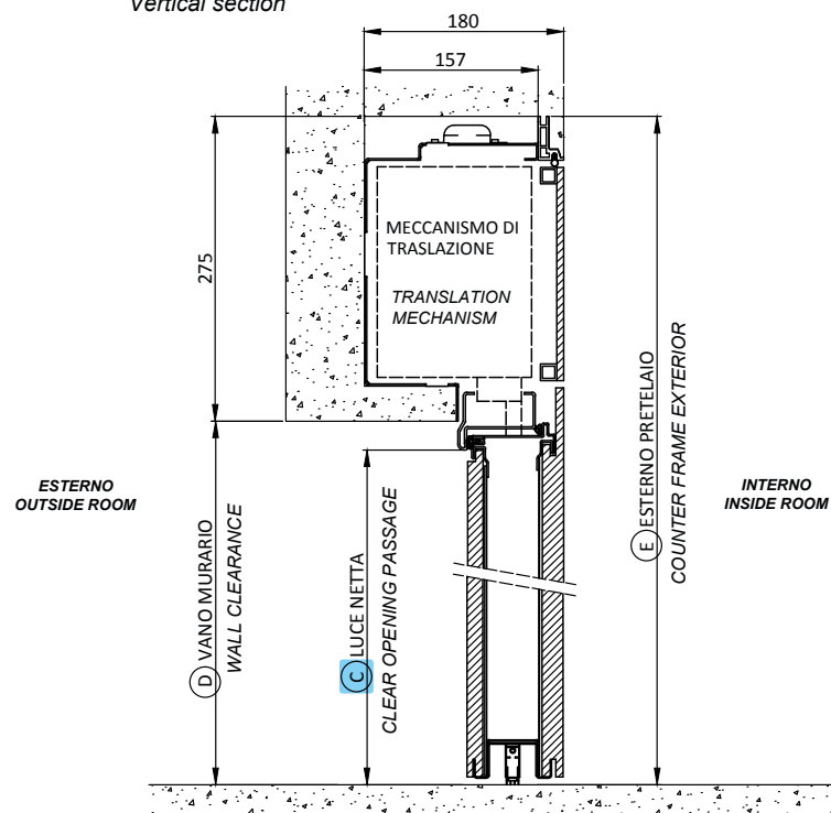
Sezione verticale C-C Vertical section
