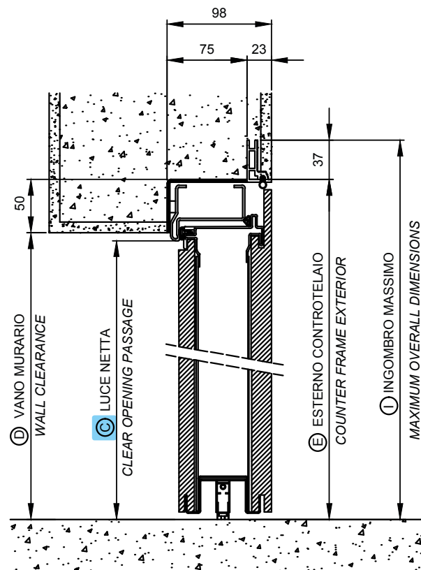
Configurazione pavimento complanare Flush floor configuration
