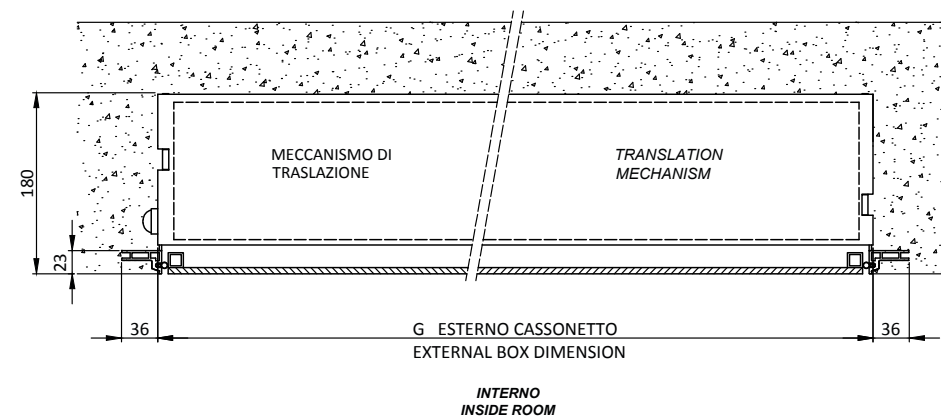
Sezione orizzontale B-B Horizontal section
