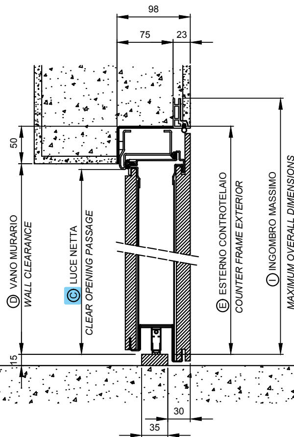
Configurazione con soglia di battuta Configuration with sill rebate
